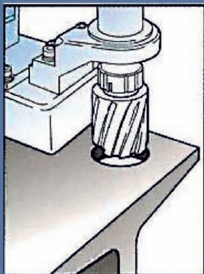
Borrning med skev utgång
