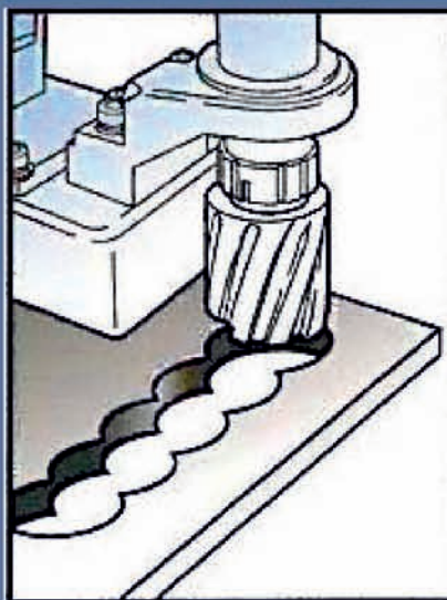
Överlapps borrning
