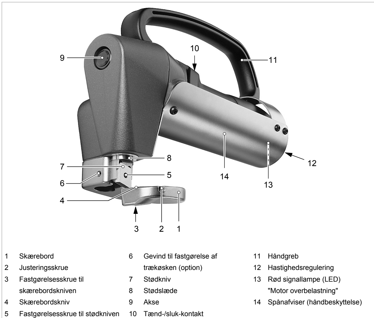
TruTool S 350
